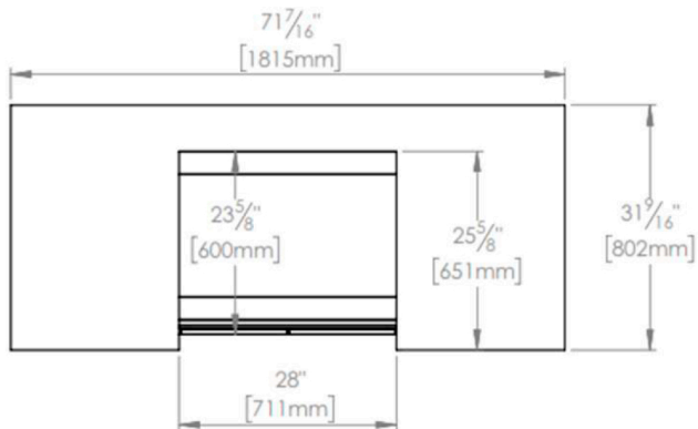
VISTA PLANTA
