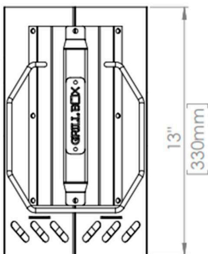
VISTA PLANTA
