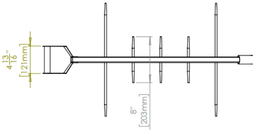
VISTA PLANTA
