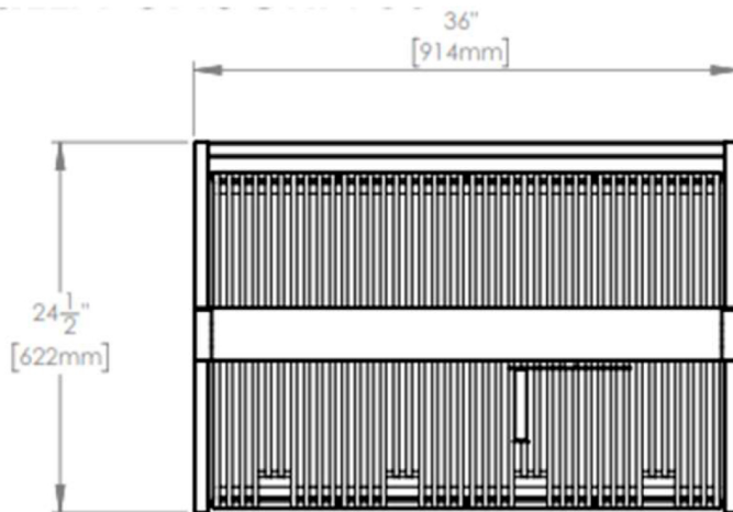
VISTA PLANTA
