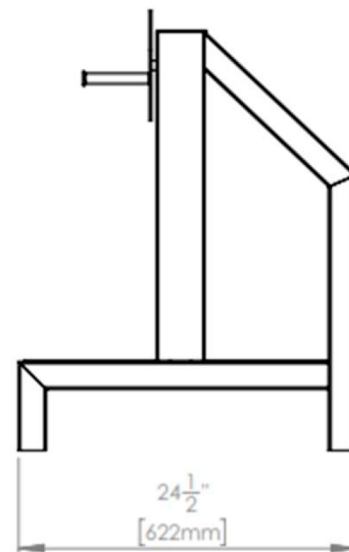
VISTA LATERAL
