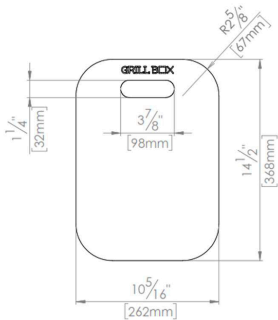
VISTA PLANTA
