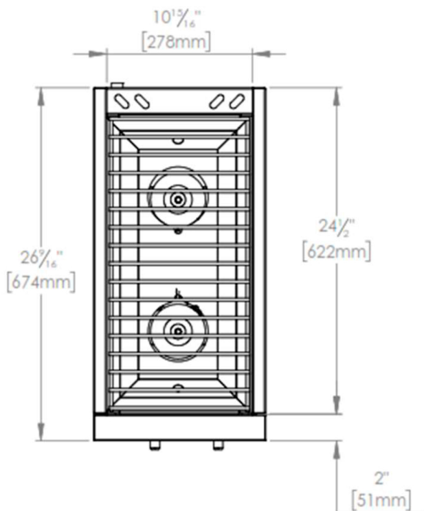
VISTA PLANTA
