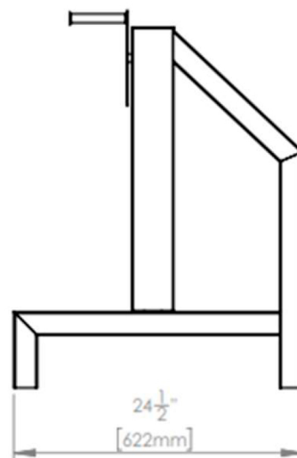
VISTA LATERAL
