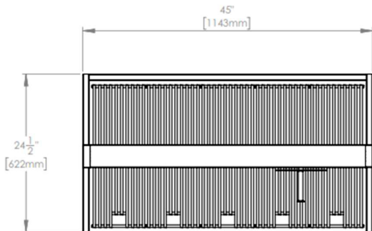
VISTA PLANTA
